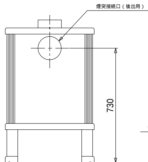
背面図
