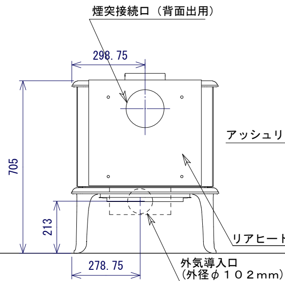
背面図
