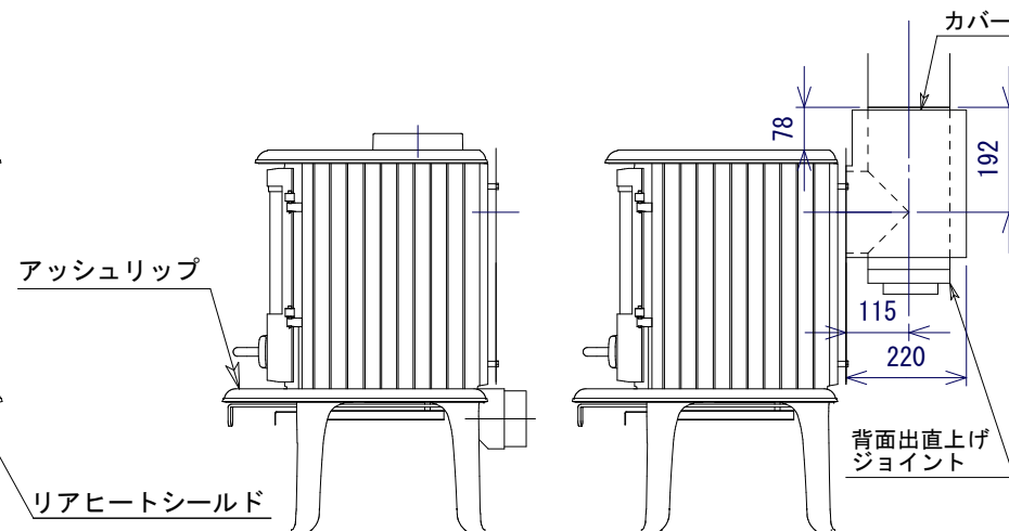
側面図
