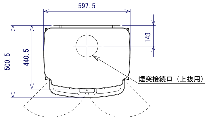
平面図
