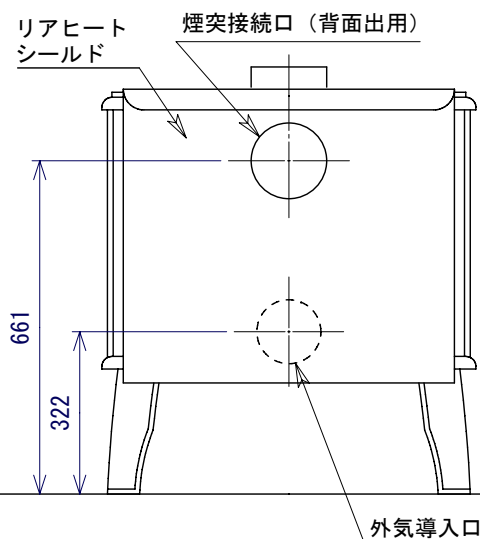
背面図
