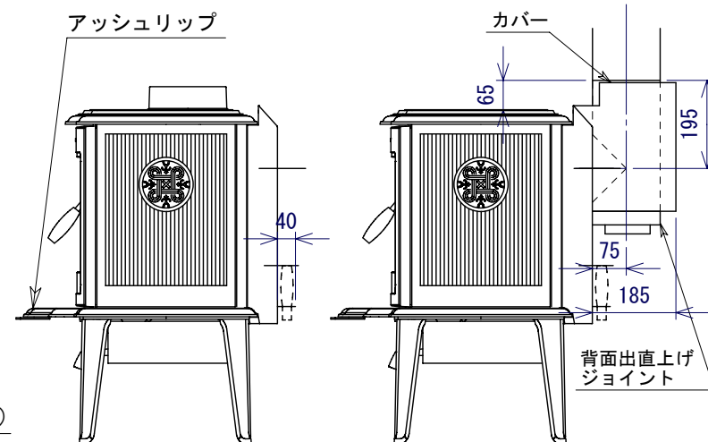
側面図
