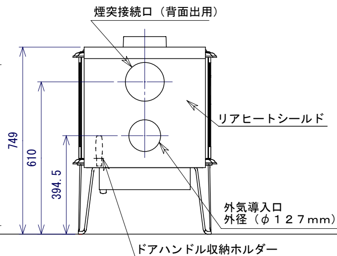
背面図
